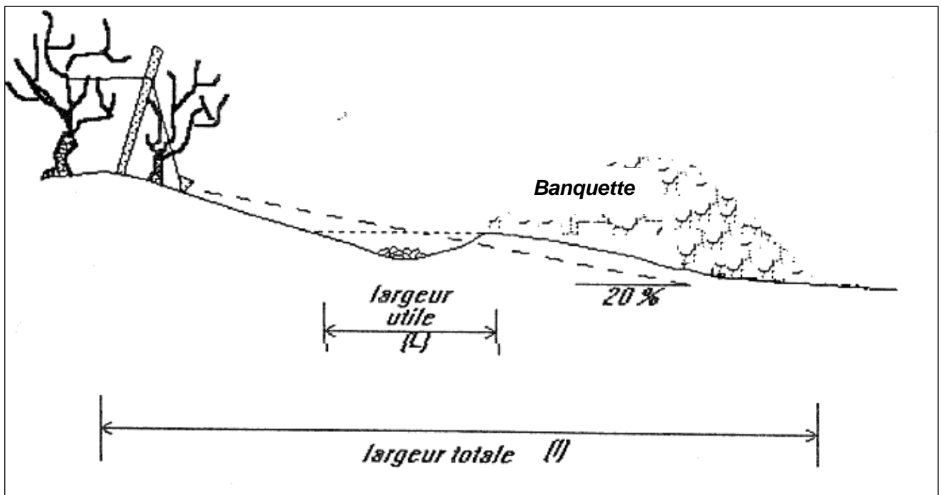
Figure 13 : Schéma de principe des canaux de contour et de drainage banquettes
