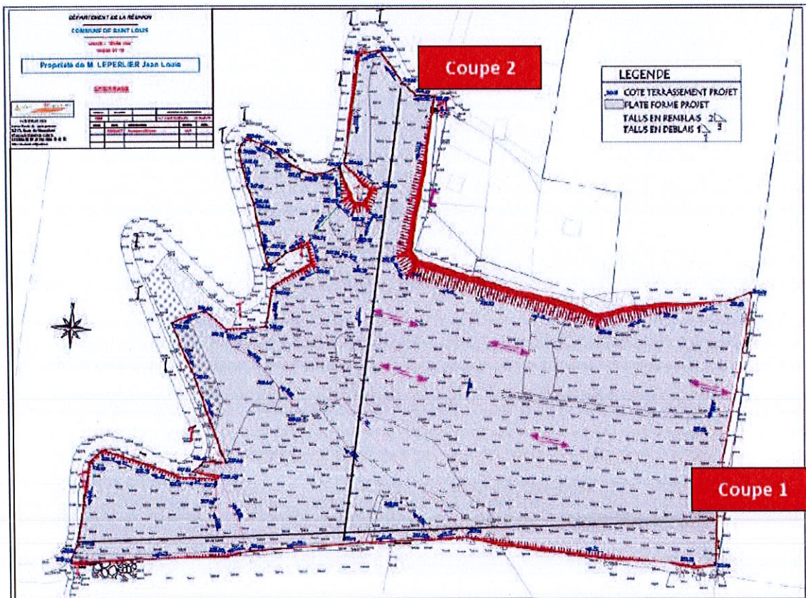
FIGURE 30 : PLAN D'AMENAGEMENT FINAL (PLATEFORMES)
